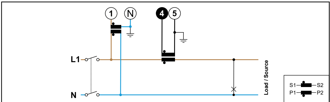
1 Phase, 2 Leiter (VT/CT-Anschluss)
