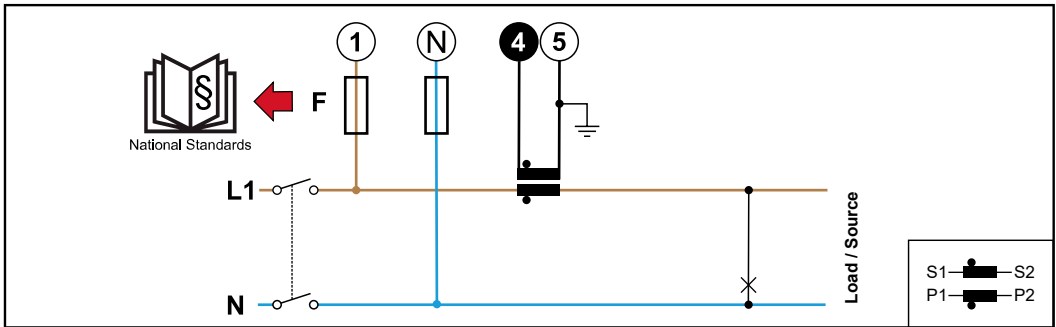
1 Phase, 2 Leiter (CT-Anschluss)
